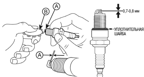
Рис. 16. Проверка межэлектродного зазора
