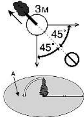
Рис. 8 Зона безопасности при валке дерева
