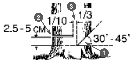
Рис. 9 Расположение запила, пропила и недопила
