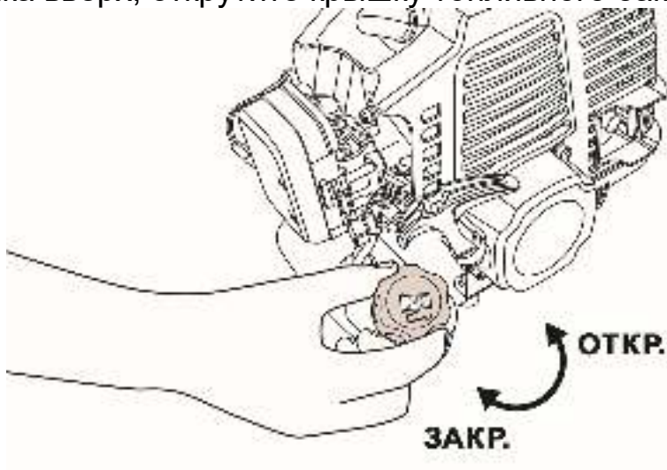
Рис. 6 Откручивание крышки топливного крана
