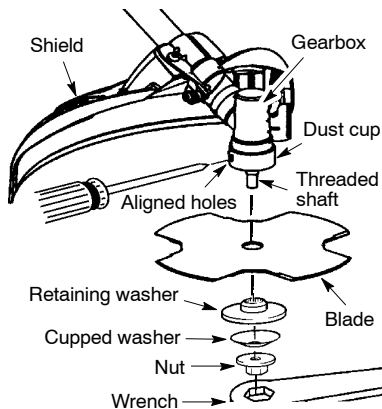
WEED BLADE
