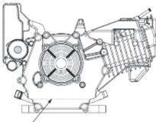
Уровень масла
