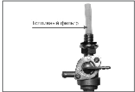
Рис. 13 Обслуживание топливного фильтра
