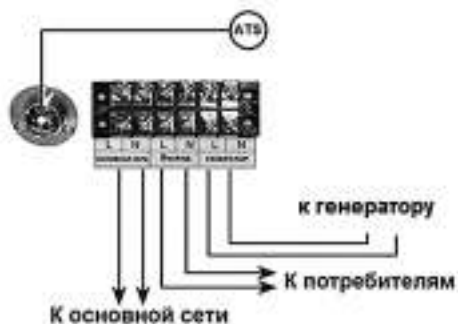
Рис. 15 Схема подключения блока ATS
