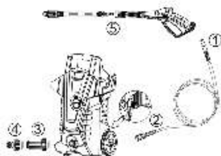
Рис. 3 Сборка аппарата
