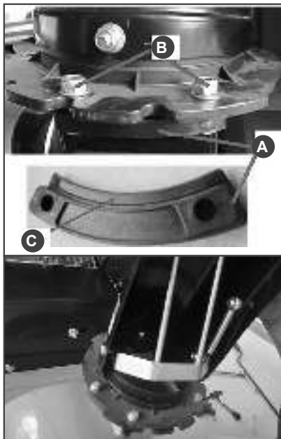
Рис. 11 Установка разгрузочного желоба
