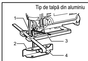
1. Bolț 2. Ghidajul riglei 3. Cheie inbus 4. Rigla de ghidare
