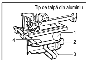
1. Buton filetat 2. Știft 3. Rigla de ghidare 4. Ghidajul riglei
