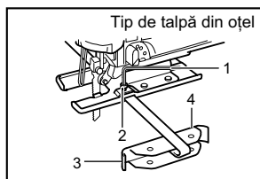
1. Cheie inbus 2. Bolț 3. Rigla de ghidare 4. Fața ghidajului
