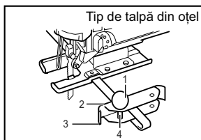
1. Buton filetat 2. Fața ghidajului 3. Rigla de ghidare 4. Știft
