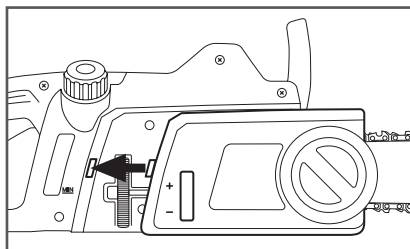
Рис. 6 Установка крышки шины
