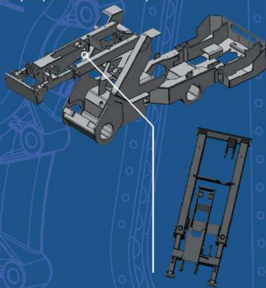
Шарнирно-сочлененная рама
