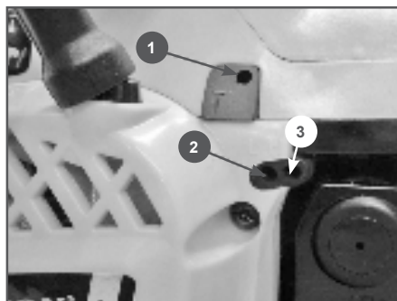
Рис. 25 Винты регулировки карбюратора 1. Винт «Т» 2. Винт «L» 3. Винт «H»
