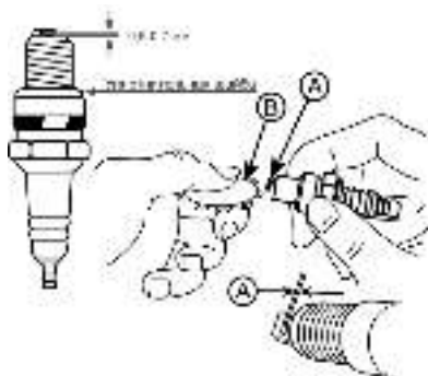
Рис. 24 Проверка зазора между электродами А – зазор В – щуп
