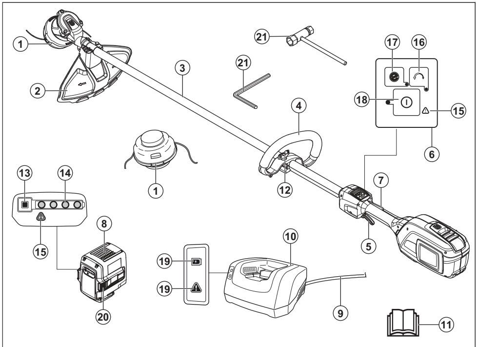
1. Головка триммера
