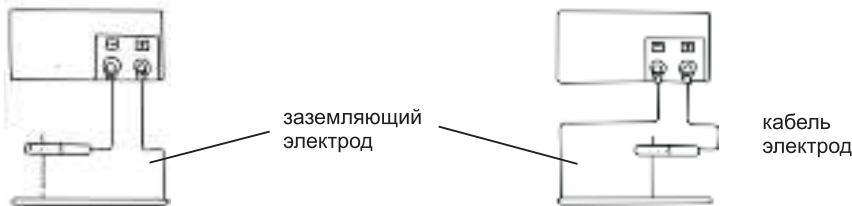
Схема сварки с прямой полярностью
