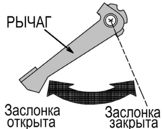
Рис. 9 Рычаг управления воздушной заслонкой IGG1200
