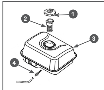
Рис. 16 Топливные фильтры
