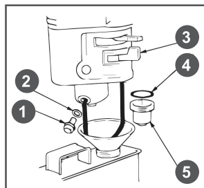
Рис. 17 Обслуживание фильтра-отстойника
